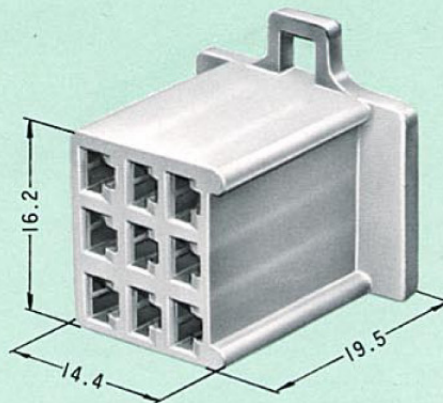
ハウジング F (6040-9111)
