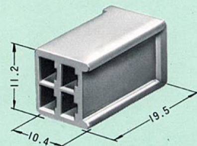
ハウジング F (6130-2340)
