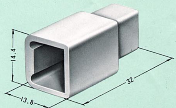
ハウジング M (6130-0540)
