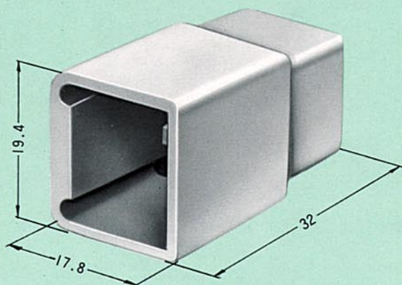
ハウジング M (6130-0590)
