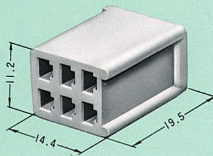
ハウジング F (6130-2360)
